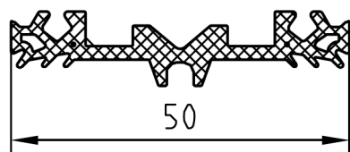
760 600 glasafdichting buiten EPDM Constructiebreedte 50/60 mm, te koop per 50 m
