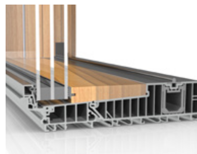
Seitenschnitt mit Verglasung der Hebe-Schiebe-Tür „HST“
