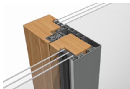
Detailschnitt mit drei Dichtungsebenen am Mittelstoß
