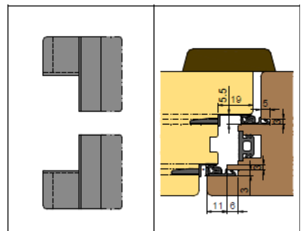
Inbouwvoorbeeld SK 300 (groef 3 mm)
